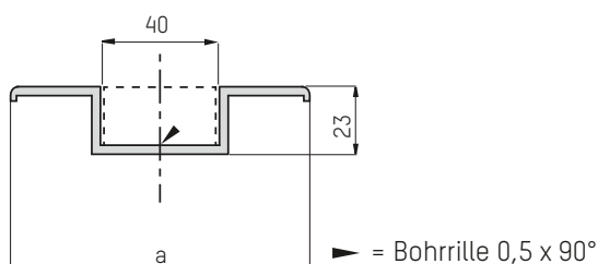
Fugenleiste 3 mm
